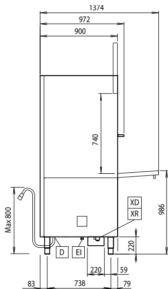
Bočna/o
