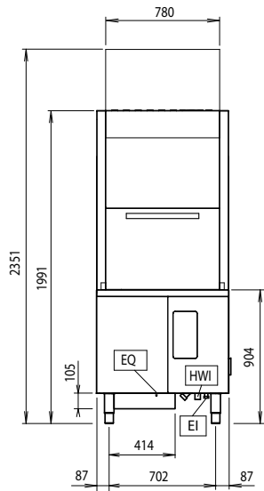
Prednja/e
